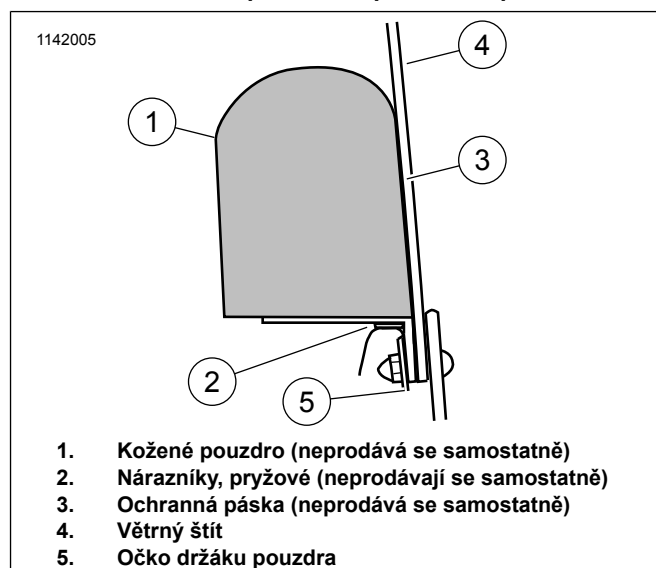
Ilustrace 2. Připevnění přichytky kapotáže, boční zobrazení
