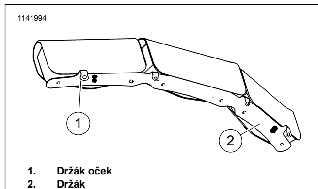
Ilustrace 1. Spodní část pouzdra kapotáže
