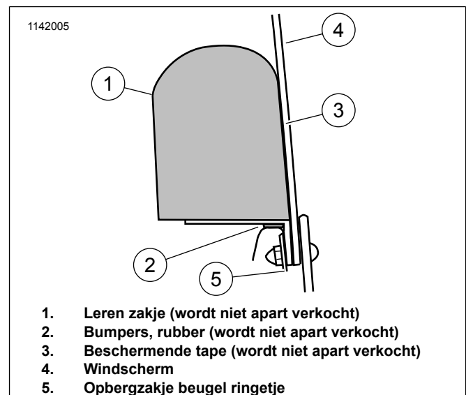
Afbeelding 2. Bevestiging voor kuipclip, zijaanzicht
