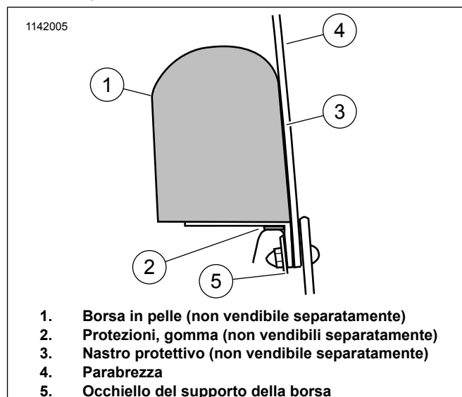
Figura 2. Accessorio a fermaglio per borsa, vista laterale
