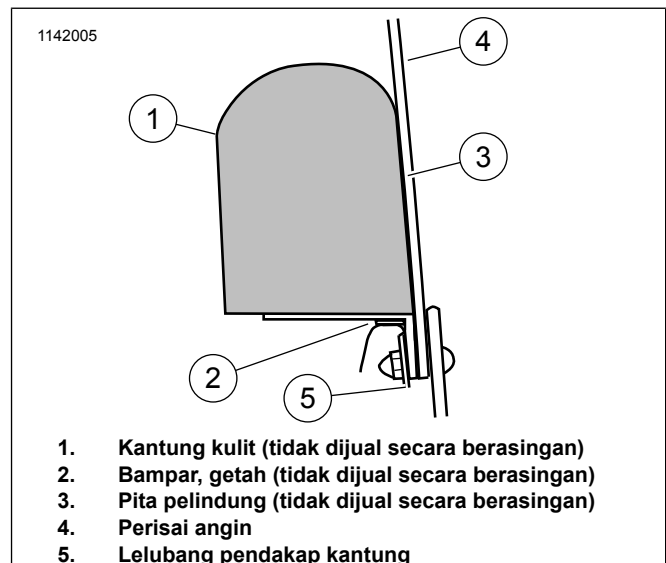
Rajah 2. Lampiran Klip Reraut, Paparan Sisi
