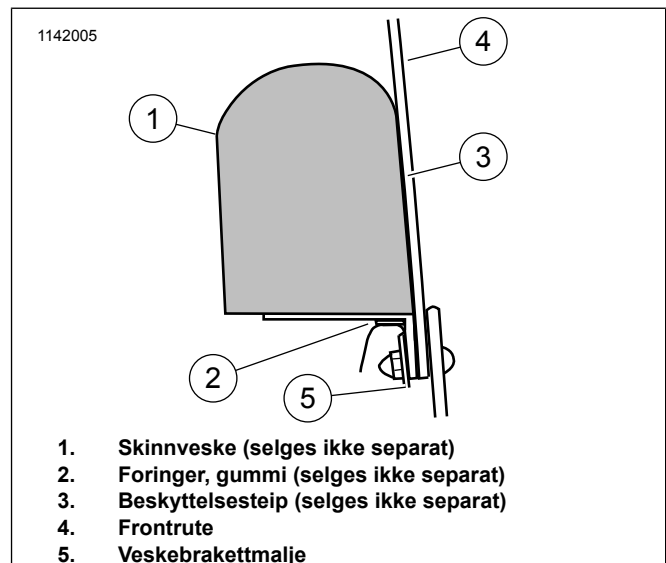
Figur 2. Kåpeklipsfeste, sidevisning
