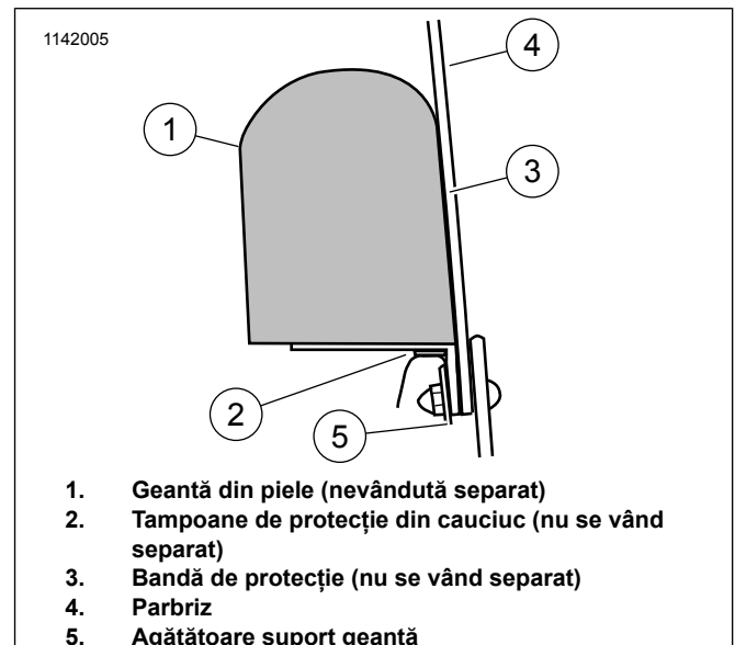
Figura 2. Fixare carenaj cu clemă, vedere laterală
