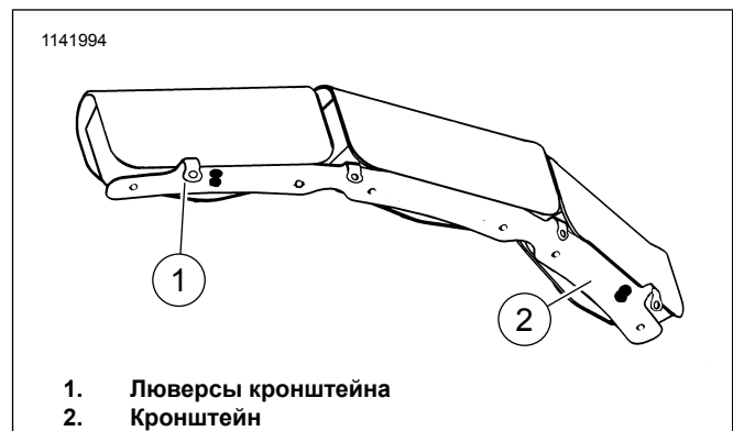
Рисунок 1. Нижняя часть сумки на обтекатель
