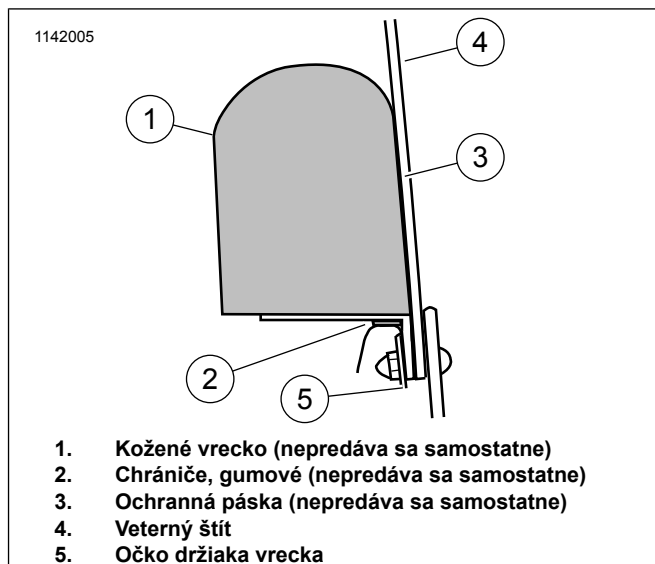
Obrázok 2. Príchytkový nástavec kapotáže, bočné zobrazenie
