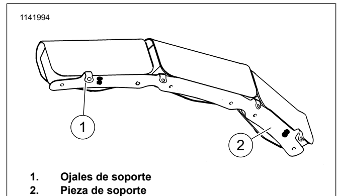
Figura 1. Parte inferior de la funda del carenado
