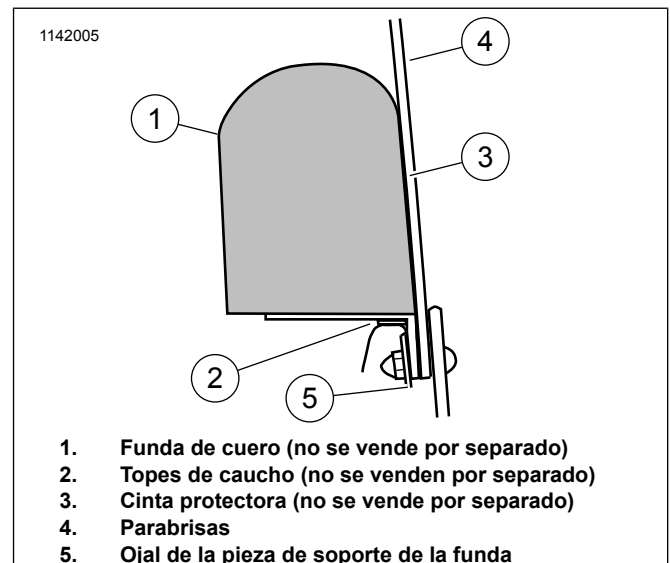
Figura 2. Accesorio de la presilla de carenado, vista lateral
