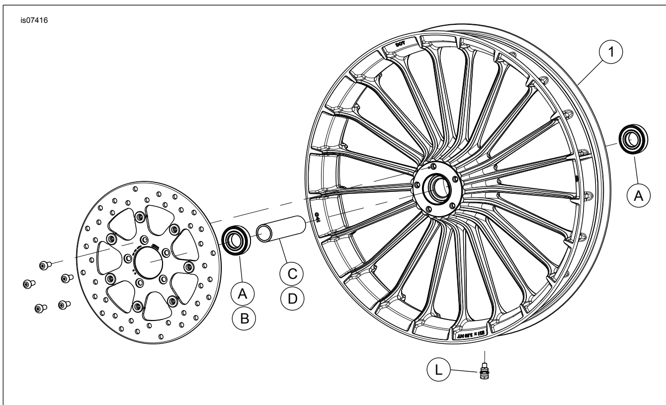
Figura 2. Componente de service: Roata din față a turbinei
