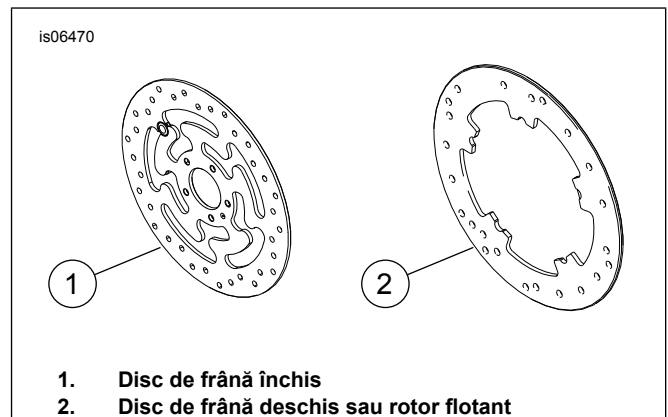
Figura 1. Stilurile discului de frână din față
