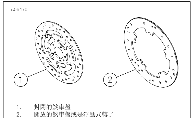
圖1. 前煞車盤樣式
