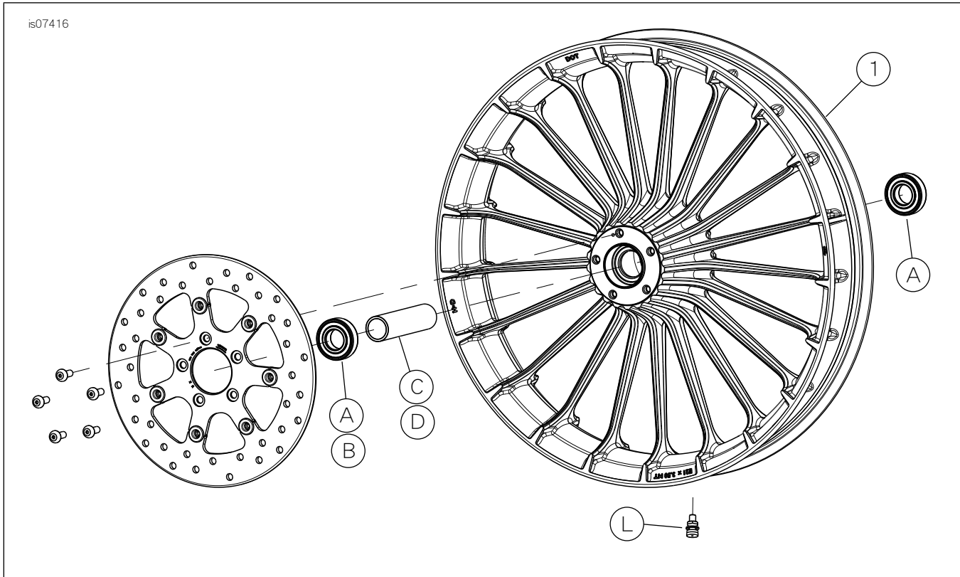
圖2。維修零件前渦輪
