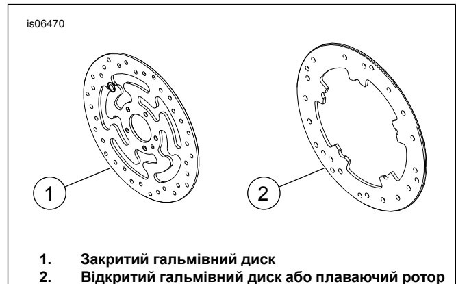
Малюнок 1. Стилі дисків передніх гальм
