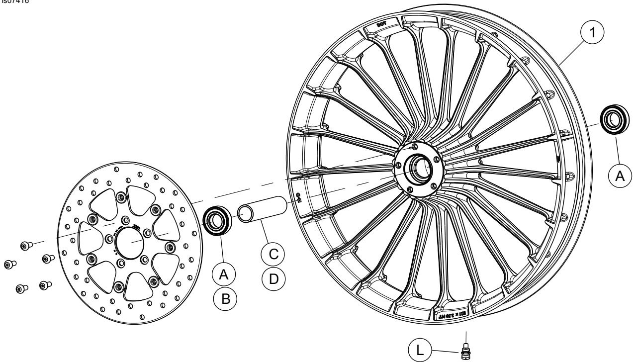
Малюнок 2. Запчастини, що обслуговуються: Переднє колесо турбіни
