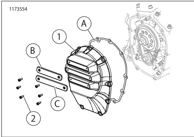
図1。Milwaukee-Eightカムカバー(標準)
