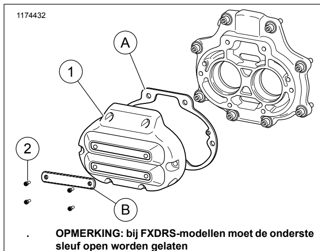
Afbeelding 1. Deksel van de versnellingsbak
