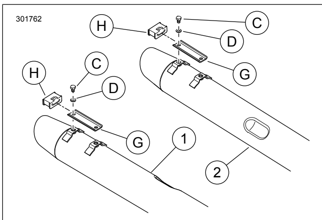
Figure 2. Support de silencieux arrière
