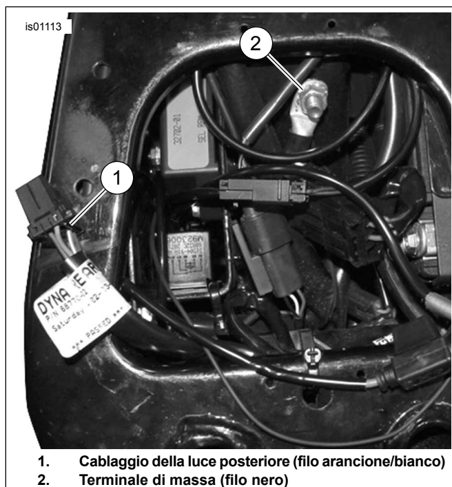
Figura 2. Collegamenti di alimentazione e a massa (modelli Dyna)
