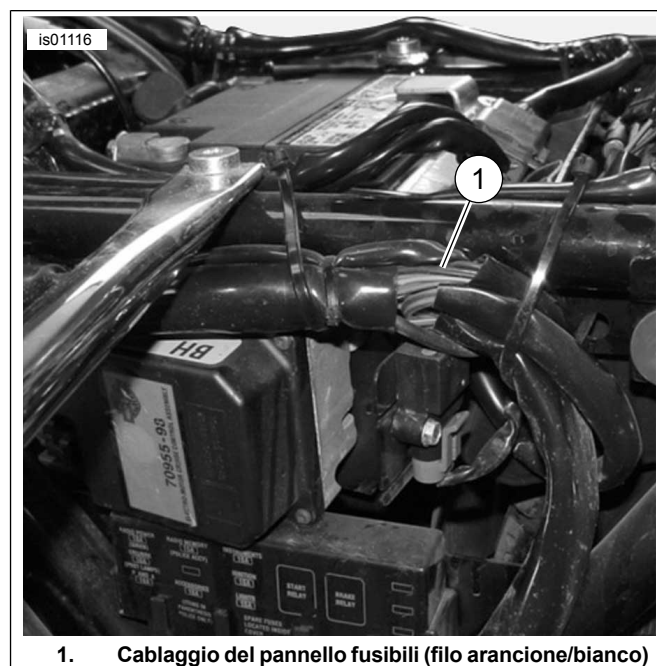
Figura 12. Cablaggio del pannello fusibili dietro il coperchio sinistro, modelli Touring fino al 2003 (è mostrato il modello FLHTCU)
