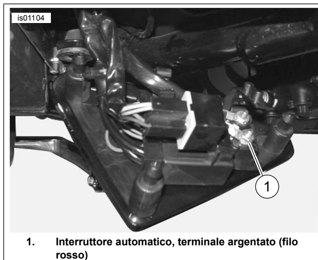
Figura 19. Interruttore automatico (modelli Sportster 2003 o anni precedenti)
