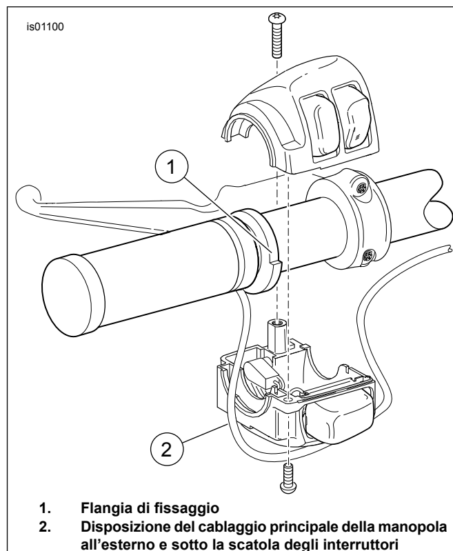
Figura 1. Manopola riscaldata (lato sinistro)
