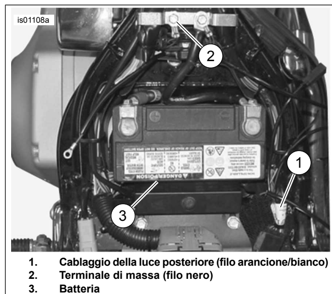
Figura 3. Collegamenti di alimentazione e a massa (modelli Softail)
