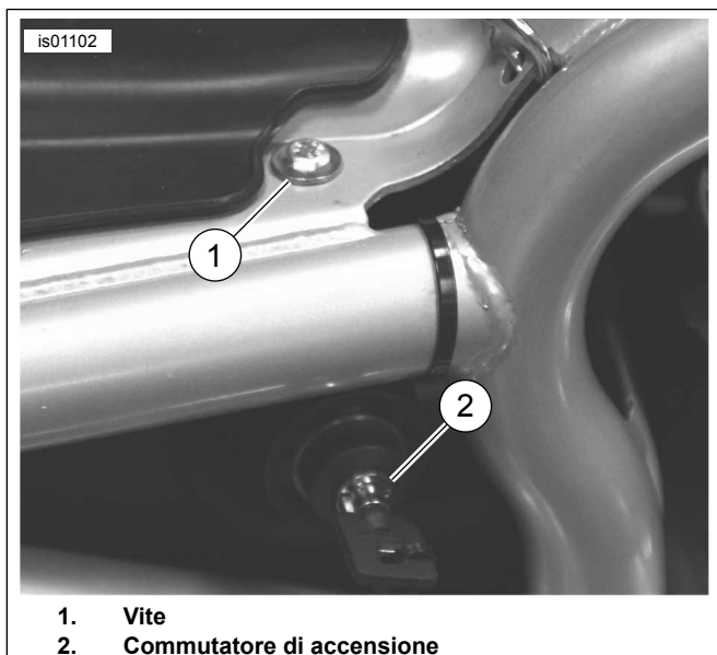
Figura 6. Collegamento di terra (modelli V-Rod 2006 e anni precedenti)
