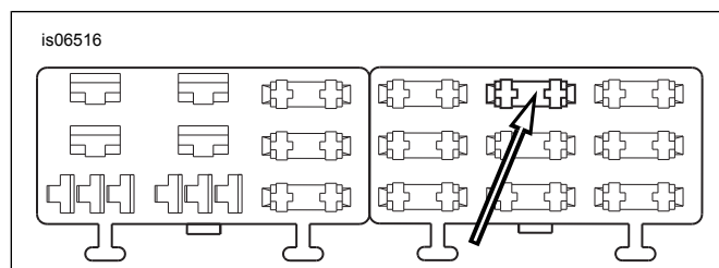
Figura 10. Cavità del pannello fusibili "P&A IGN" (modelli Softtail dal 2004 al 2010)
