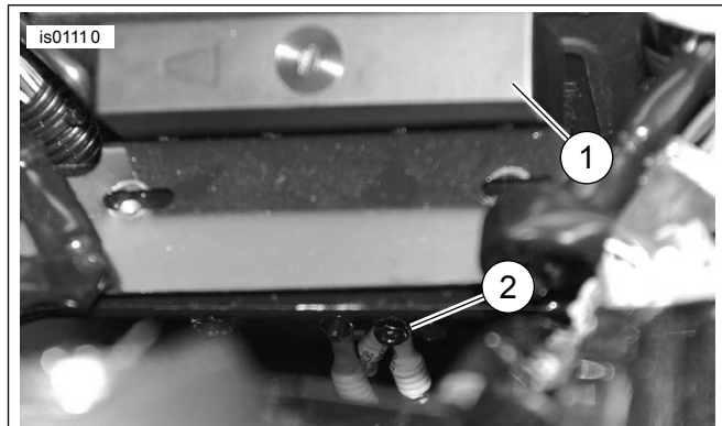
1. Caja de fusibles 2. Disyuntor, terminal plateado (cable rojo)
