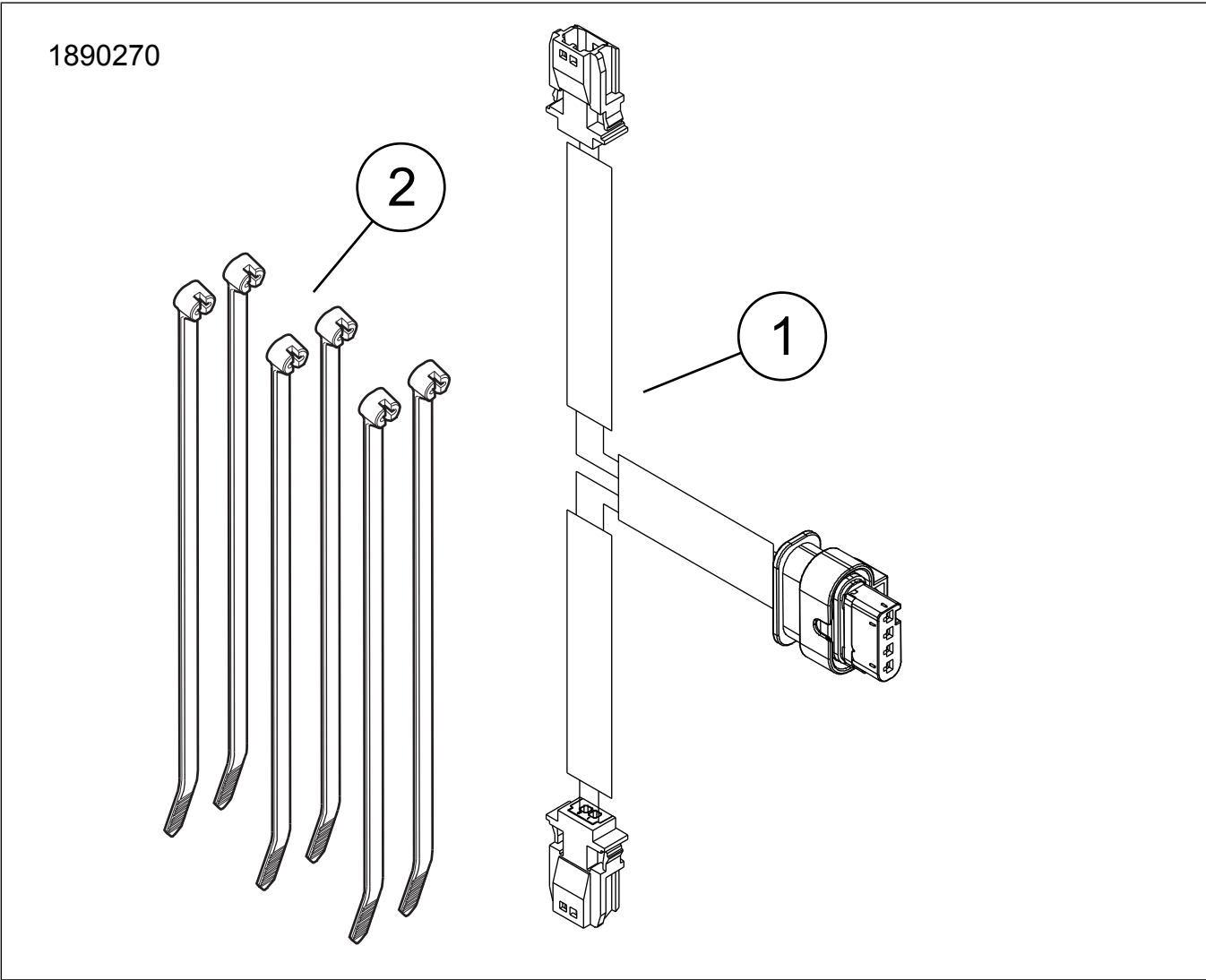
Figura 1. Contenido del kit: ARNÉS DE CABLEADO DE LAS LUCES PARA NIEBLA LED ESTILO BALA
