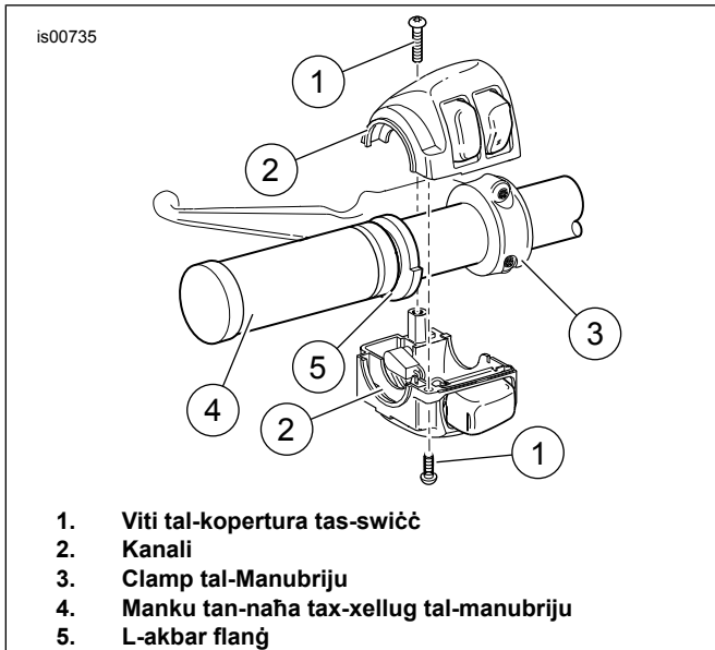
Figura 1. Kopertura tas-Swiċċ tan-Naħa tax-Xellug tal-Munbriju
