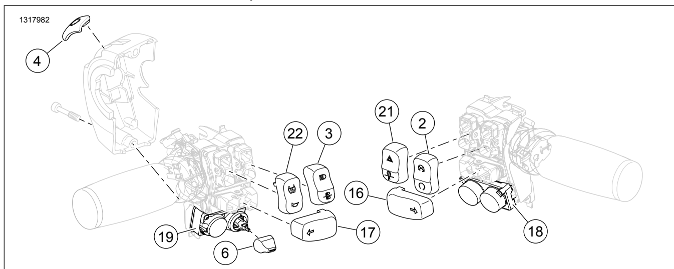
Joonis 5. Varuosad komplektile 71500517: Juhtraua lülite kroomitud lülitikatted
