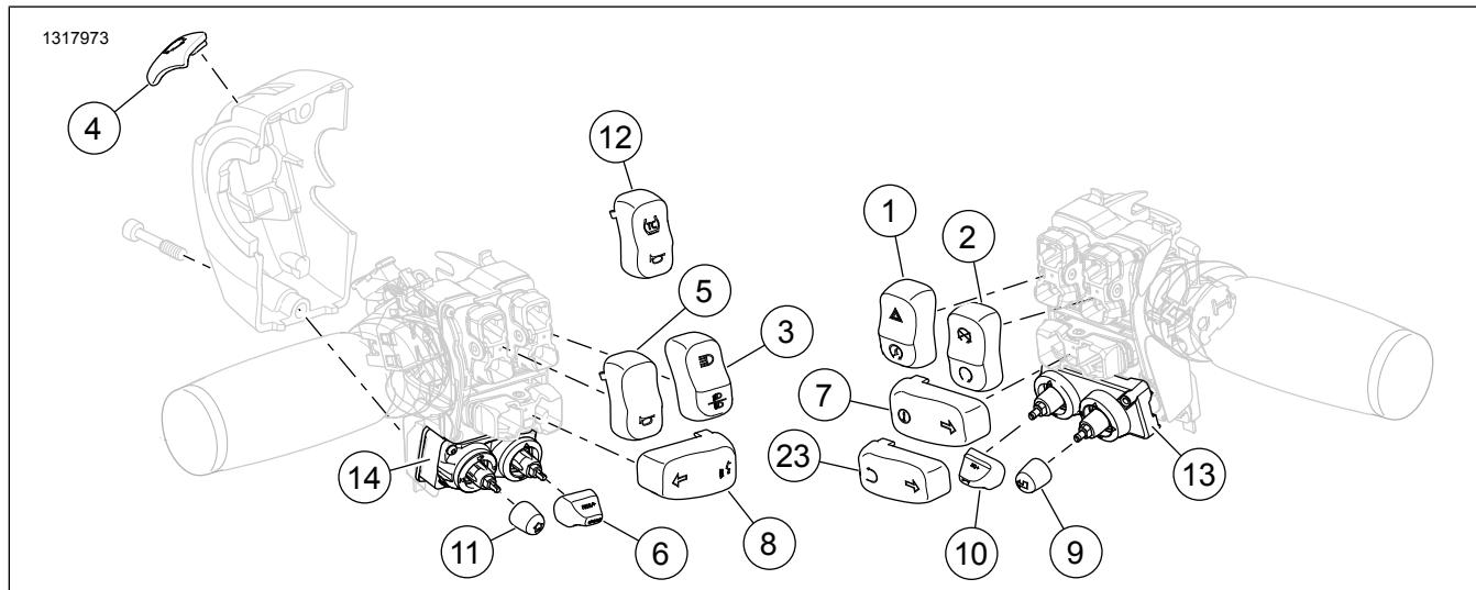
Joonis 1. Varuosad komplektile 71500228C: Juhtraua lülite kroomitud lülitikatted
