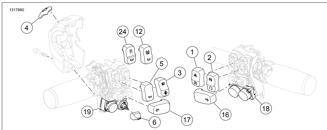
Joonis 3. Varuosad komplektile 71500186A: Juhtraua lülite kroomitud lülitikatted
