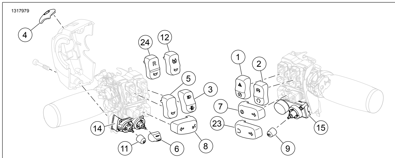
Joonis 2. Varuosad komplektile 71500187C: Juhtraua lülite kroomitud lülitikatted
