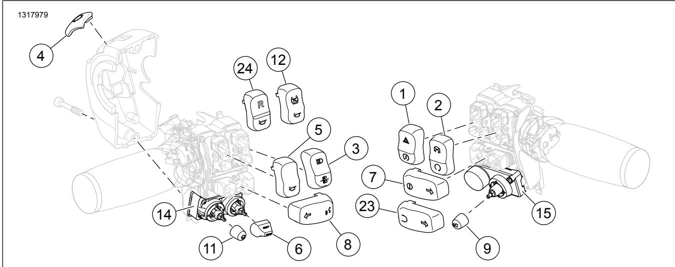
Şekil 2. 71500187C için Servis Parçaları: Krom Gidon Anahtar Başlığı Kitleri
