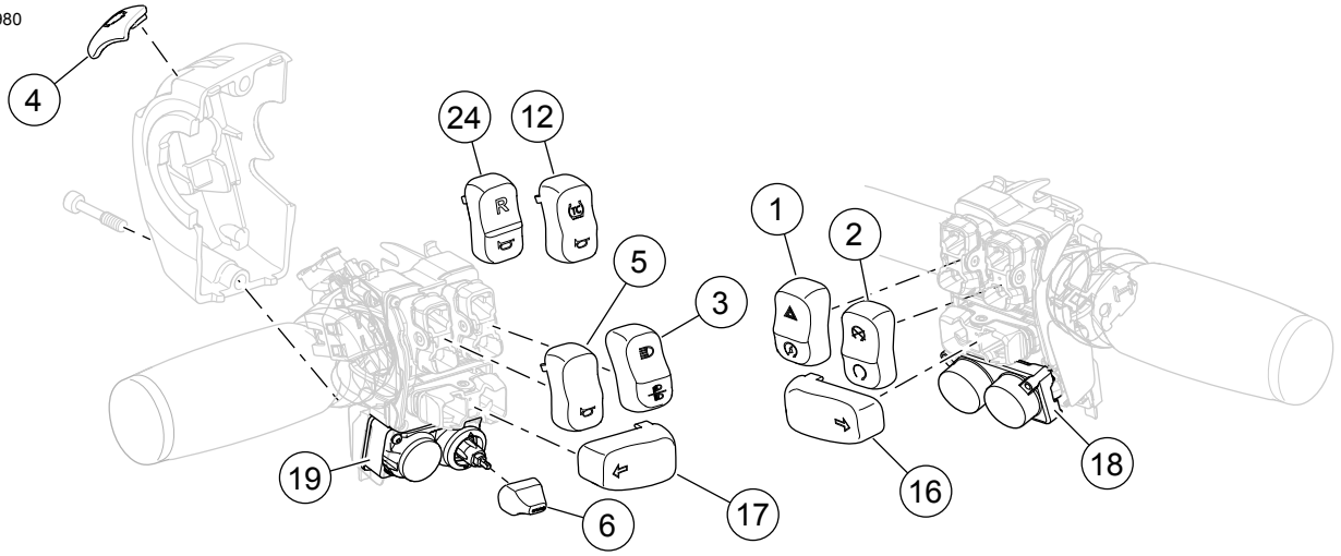
Şekil 3. 71500186A için Servis Parçaları: Krom Gidon Anahtar Başlığı Kitleri
