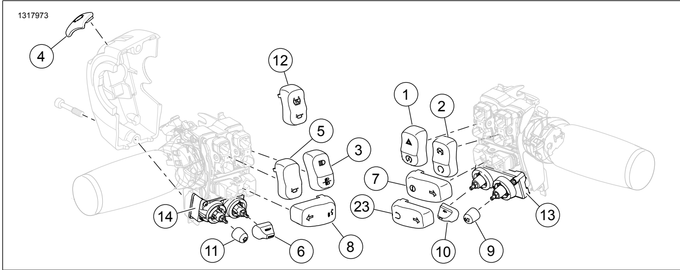
Şekil 1. 71500228C için Servis Parçaları: Krom Gidon Anahtar Başlığı Kitleri
