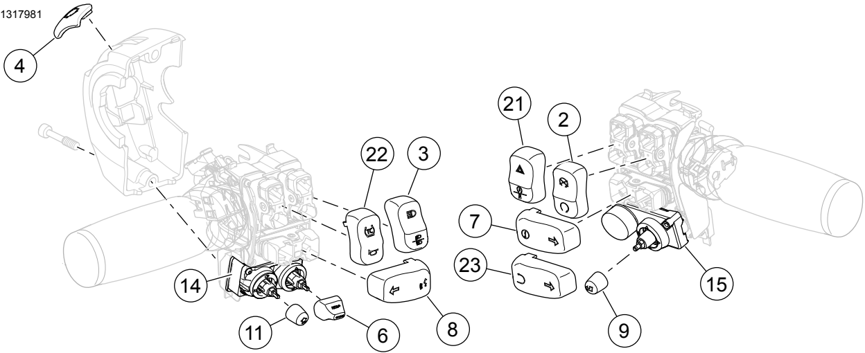
Şekil 4. 71500515 için Servis Parçaları: Krom Gidon Anahtar Başlığı Kitleri
