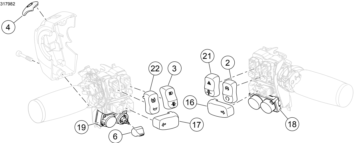
Şekil 5. 71500517 için Servis Parçaları: Krom Gidon Anahtar Başlığı Kitleri
