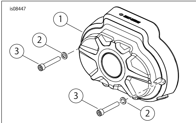
図2。バーストランスミッションサイドカバー(キット34800026用)
