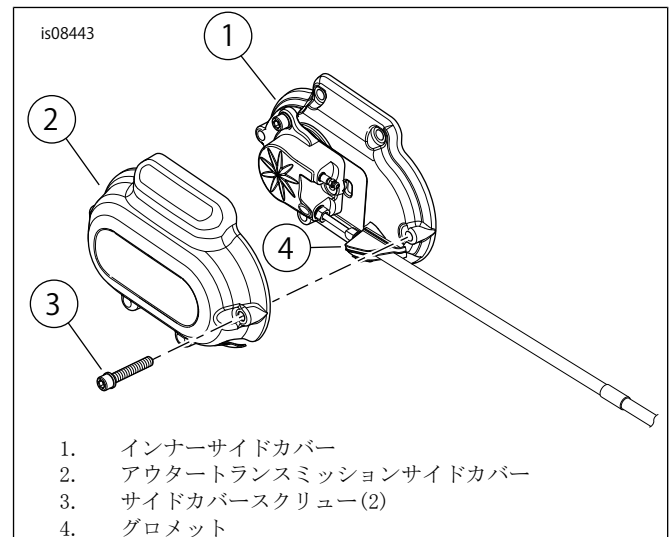
図1。トランスミッションサイドカバー
