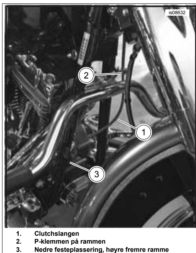
Figur 8. Lav føring av clutchvæskeslange (Softtail-modeller)
