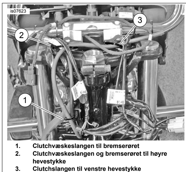
Figur 1. Slangene for clutch- og bremsvæske, modeller med kåpe (kåpe fjernet av visuelle årsaker)
