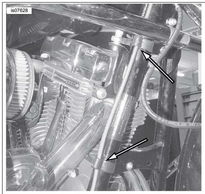
Figur 4. Plassering for klemmer på nedadgående rammerør, modeller med kåpe
