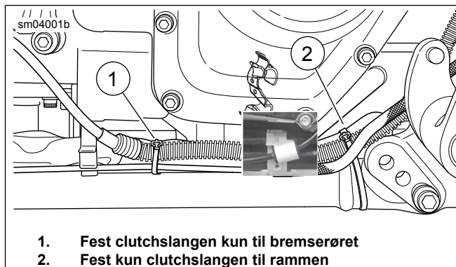
Figur 2. Plasseringen av kabelstroppene til clutchvæskeslangene
