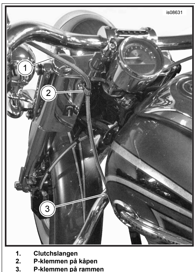
Figur 7. Høy føring av clutchvæskeslange (Softtail-modeller)
