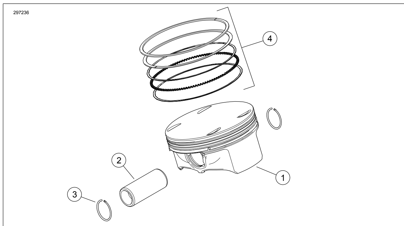
Εικόνα 1. Ανταλλακτικά: Κιτ εμβόλων 128/131 μεγάλης διαμέτρου Screamin' Eagle
