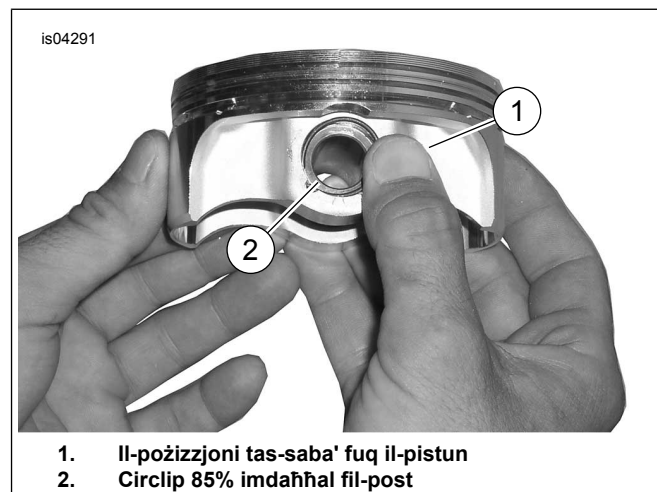
Figura 4. Installa s-circlip
