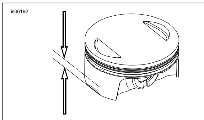
Figura 2. 0.5 pulzier (12.7 mm)
