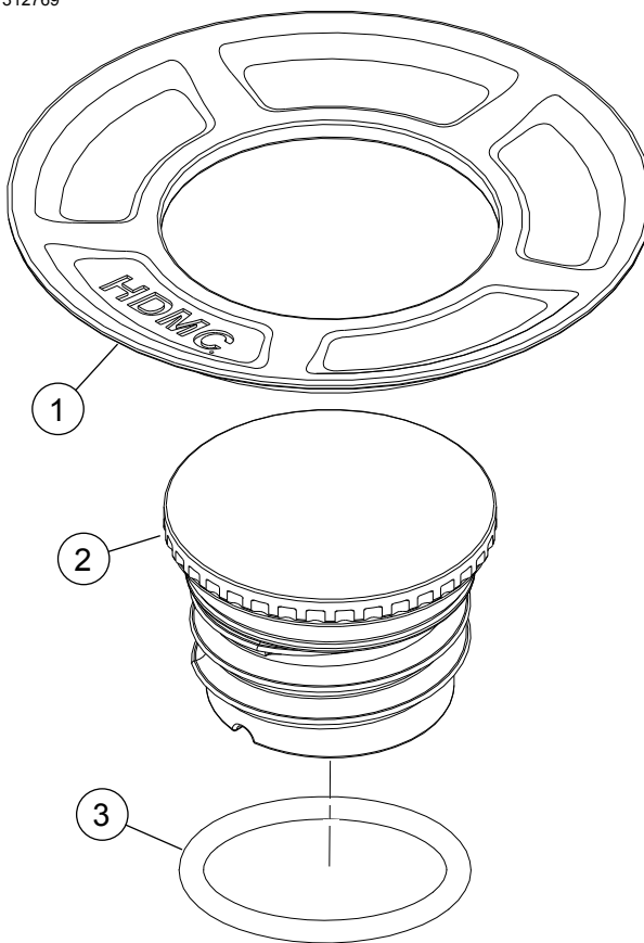
Figure 2. Pièces de rechange : Kit de bouchon de carburant encastré
