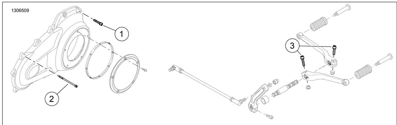
Figure 1. Contenu du kit : Composants de carter de chaîne primaire Touring
