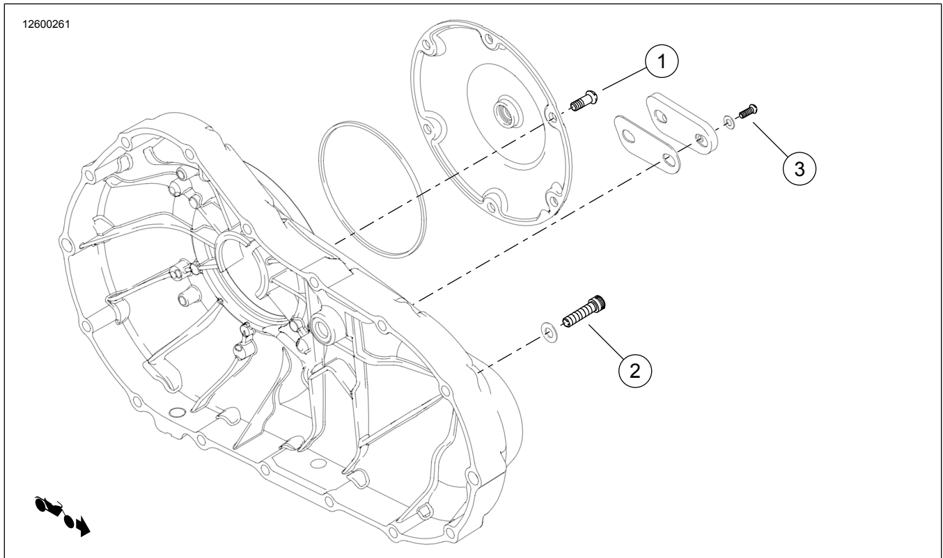
Figure 1. Contenu du kit : Composants de trappe d'embrayage et de carter de chaîne primaire XL
