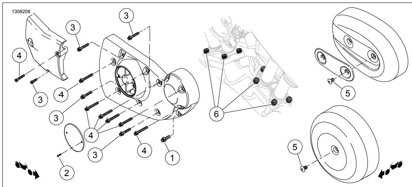
Figura 1. Kontenut tal-Kit: Komponenti tal-Cover tal-Cam
