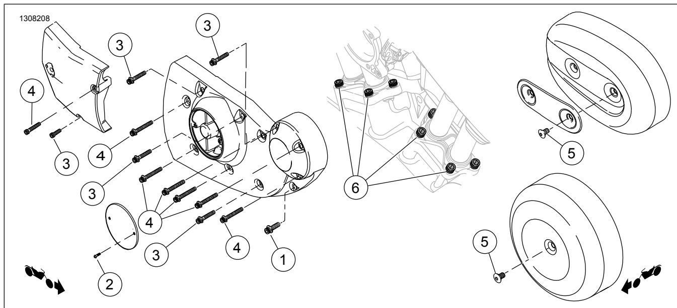
Obrázok 1. Obsah súpravy: Súčasti súpravy krytu vačky XL
