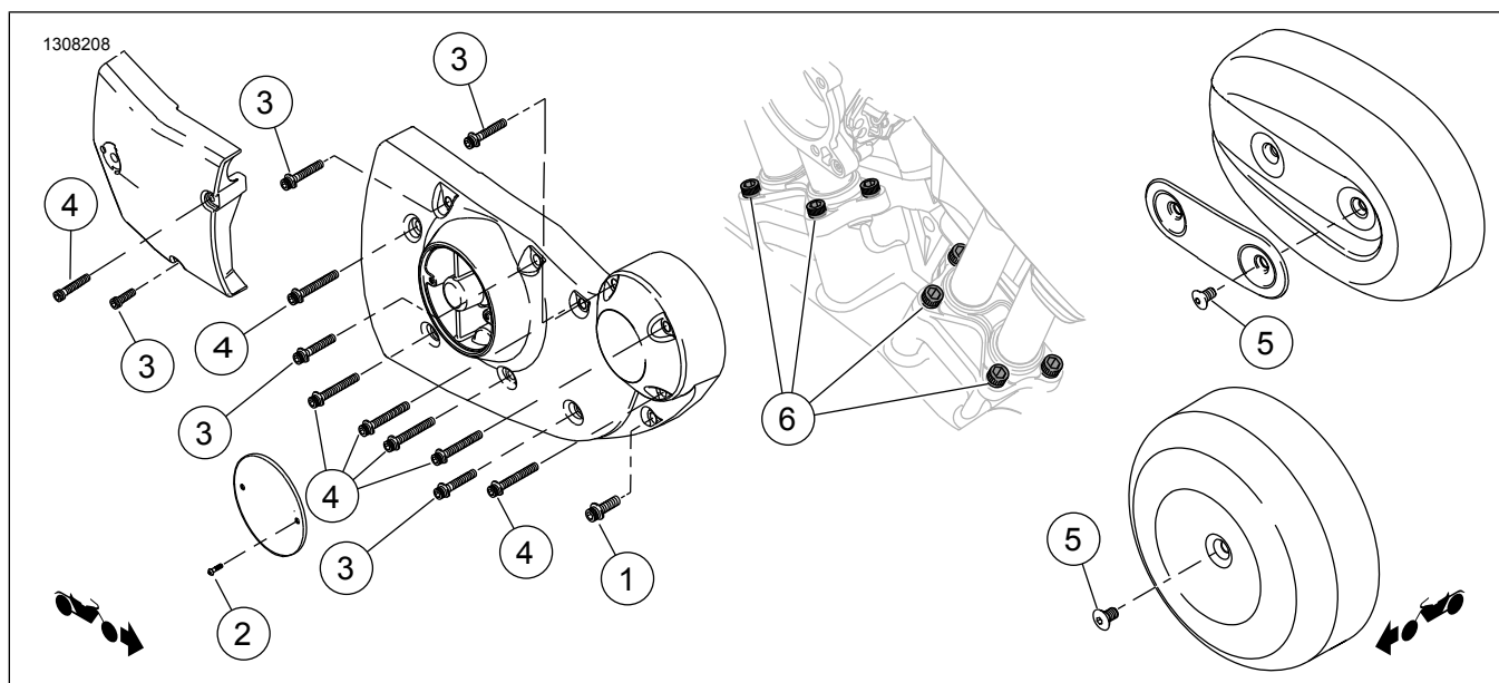
Малюнок 1. Вміст комплекту: Компоненти кришки ексцентрикового механізму XL
