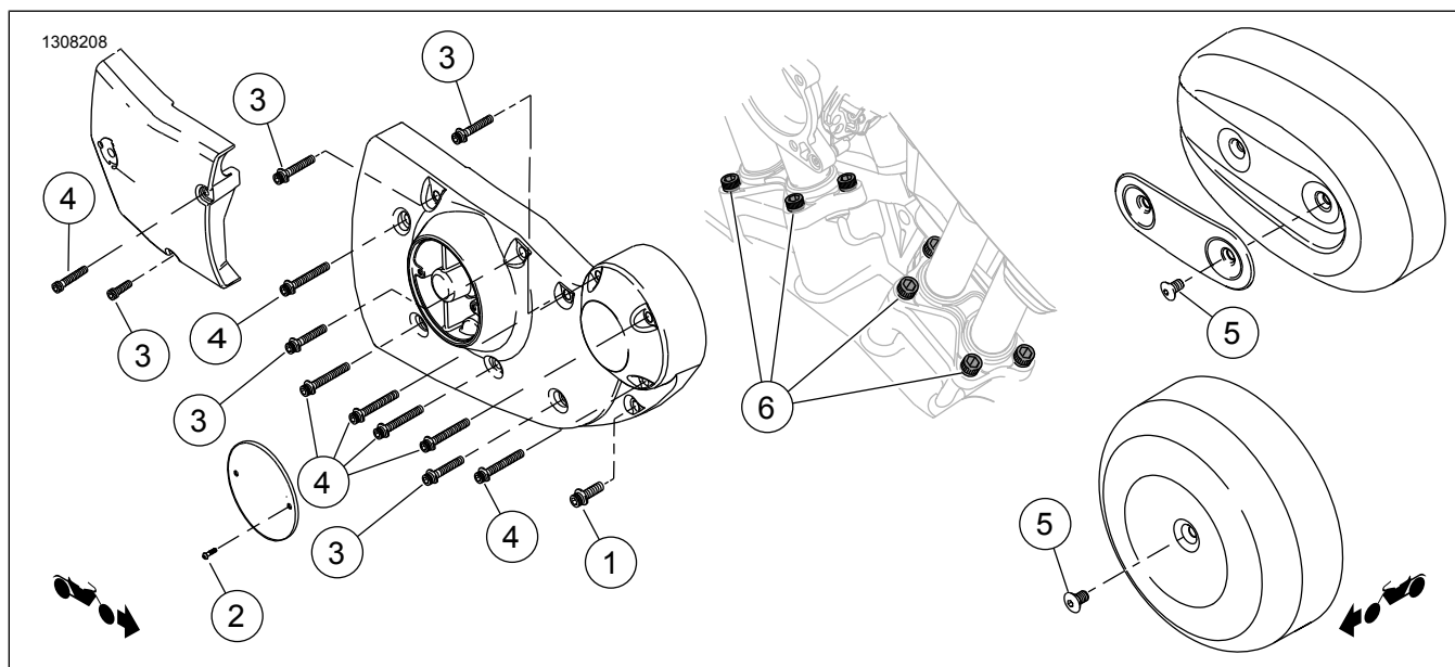
Figur 1. Sættets indhold: Dele til forspændingsdæksel
