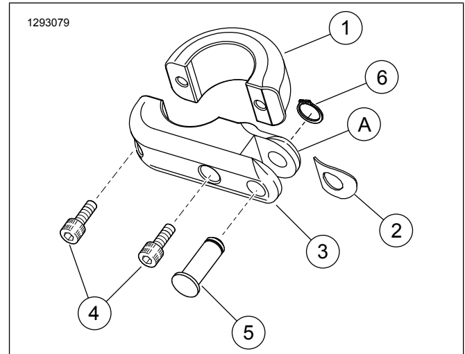
図1。交換用パーツ: エンジンガード・フットペグビレット固定キット
