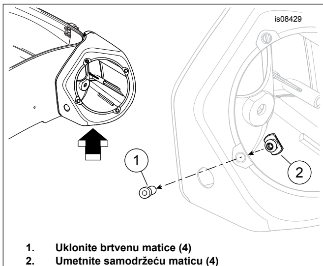
Slika 1. Uklanjanje i zamjena matica kućišta stražnjih zvučnika
