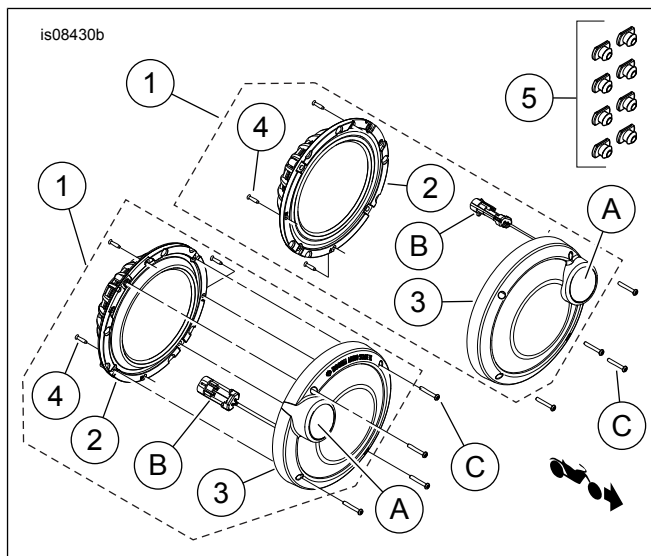
Slika 2. Servisni dijelovi, komplet stražnjeg zvučnika BOOM! Audio Stage II
