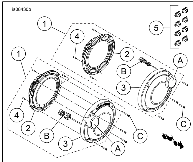
Εικόνα 2. Ανταλλακτικά, Κιτ πίσω ηχείου BOOM! AUDIO Σταδίου II
