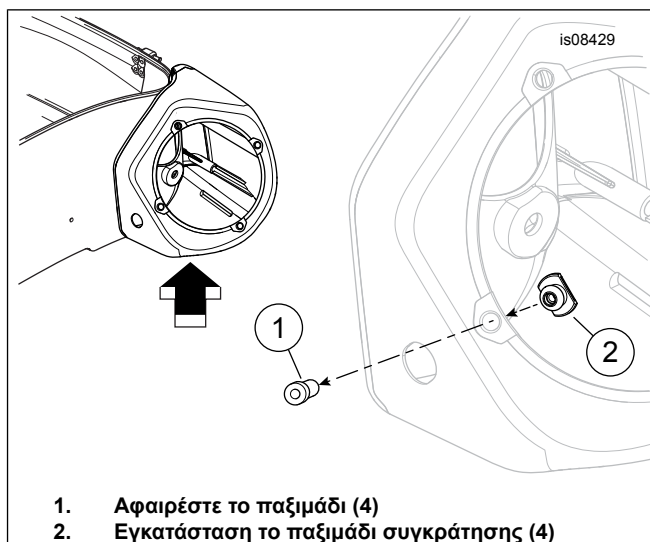
Εικόνα 1. Αφαιρέστε και αντικαταστήστε τα παξιμάδια του περιβλήματος πίσω ηχείου
