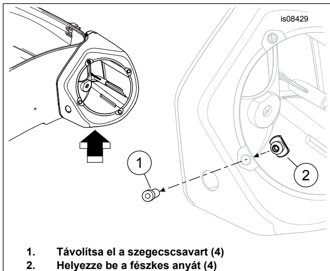
Ábra 1. Távolítsa el és cserélje ki a hátsó hangszóródoboz anyáit
