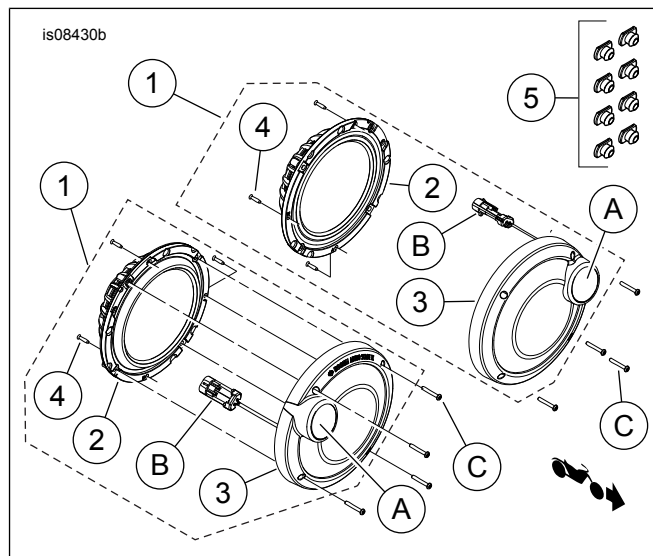
Ábra 2. Szervizalkatrészek, Boom! Audio Stage II hátsó hangszóró készlet
