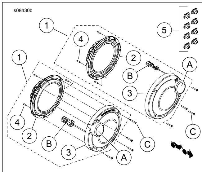
Figur 2. Servicedeler, sett for bakre høyttaler i BOOM! Audio Stage II
