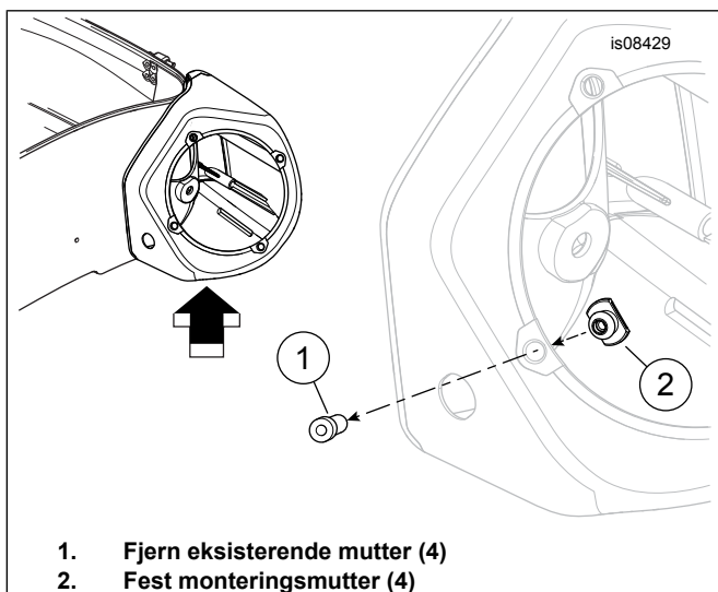
Figur 1. Fjern og erstatt mutrene til bakre høyttalerkabinett.
