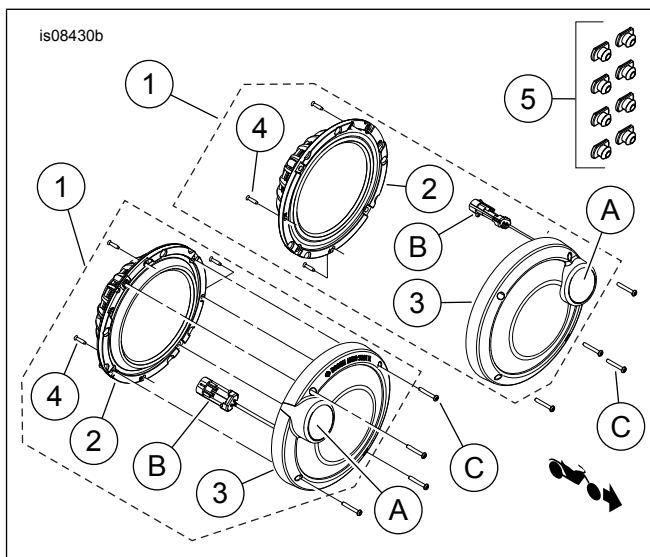
Figura 2. Piese de schimb, Kit difuzor spate BOOM! Audio etapa II
