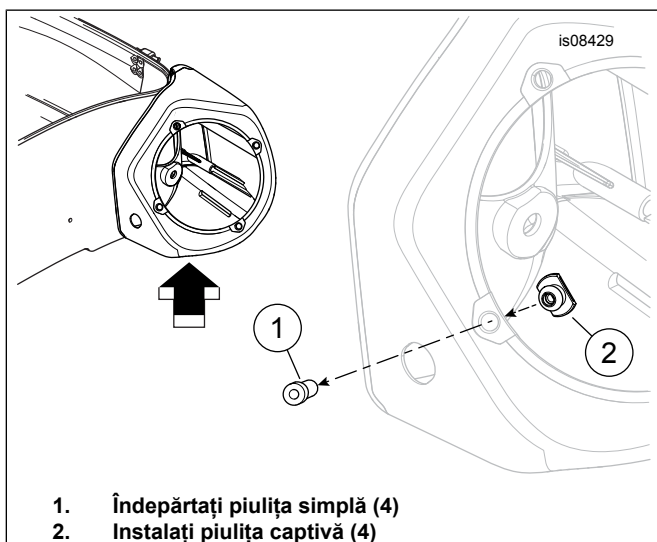
Figura 1. Scoaterea și înlocuirea piulițelor incintei difuzorului din spate
