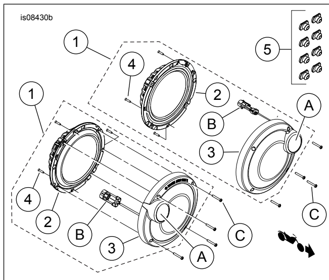
Obrázok 2. Servisné diely, súprava zadných reproduktorov BOOM! Audio Stage II
