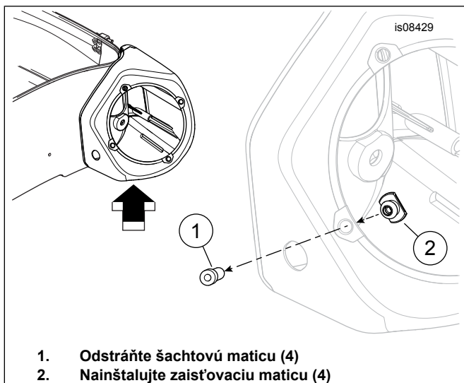
Obrázok 1. Odstráňte a vymeňte skrutky zadného krytu reproduktora
