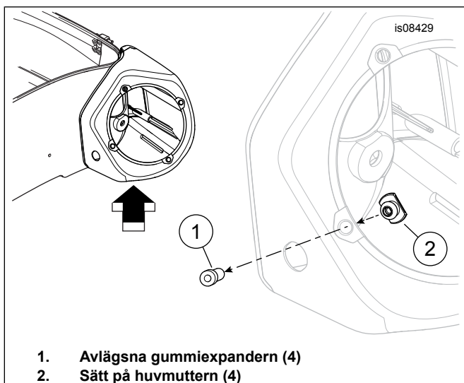
Figur 1. Avlägsna och ersätt muttrarna till den bakre högtalarinfattningen
