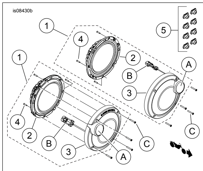
Малюнок 2. Запчастини, що обслуговуються, комплект задніх динаміків BOOM! Audio Stage II
