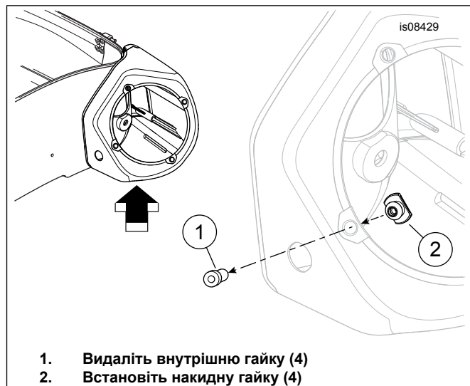
Малюнок 1. Видаліть і замініть гайки корпусу заднього динаміка
