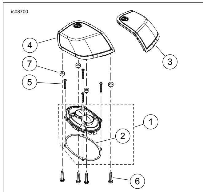
Pav 3. Prižiūrimos dalys, „Boom! Audio Stage II“ balnakrepšių garsiakalbių rinkinys
