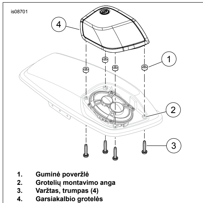
Pav 2. Grotelių montavimas
