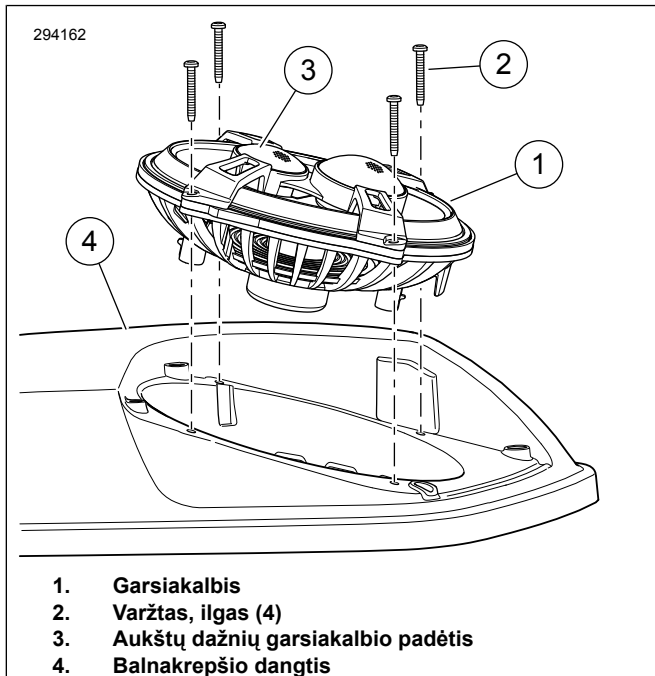
Pav 1. Garsiakalbio padėtis
