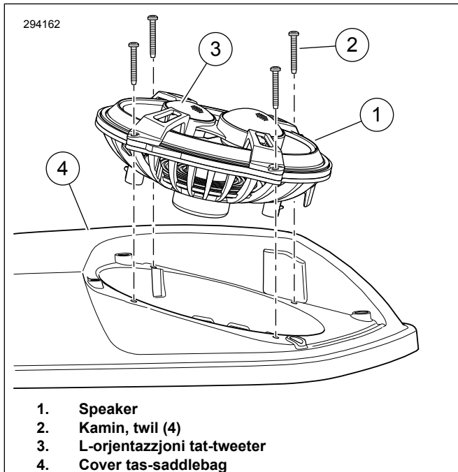
Figura 1. L-orjentazzjoni tal-ispiker
