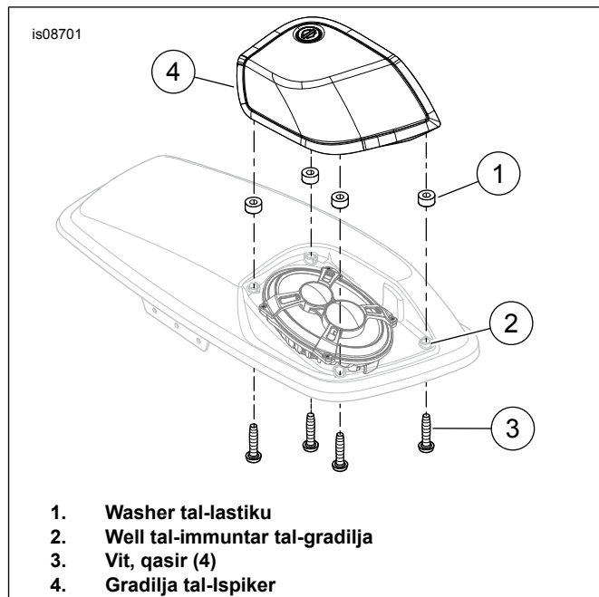
Figura 2. Installazzjoni tal-Gradilja
