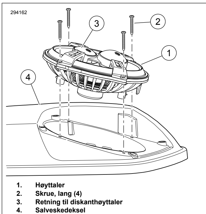
Figur 1. Høytallerretning
