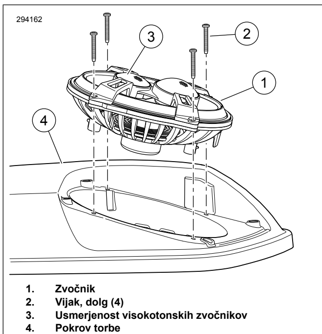
Slika 1. Usmerjenost zvočnikov
