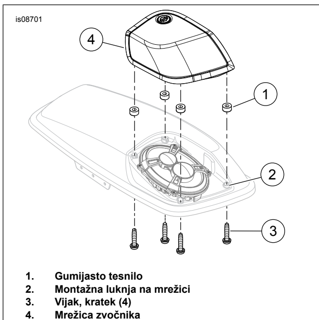
Slika 2. Namestitev mrežice
