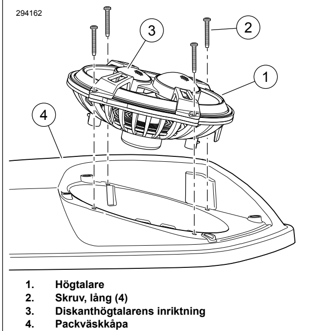
Figur 1. Högtalarens inriktning
