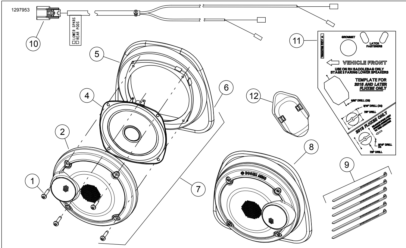
Kuva 4. Varaosat, tuulisuojan alakatteen kaiuttimet
