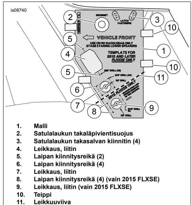
Kuva 3. Oikean satulalaukun leikkaus ja valjaiden asennus-poraus
