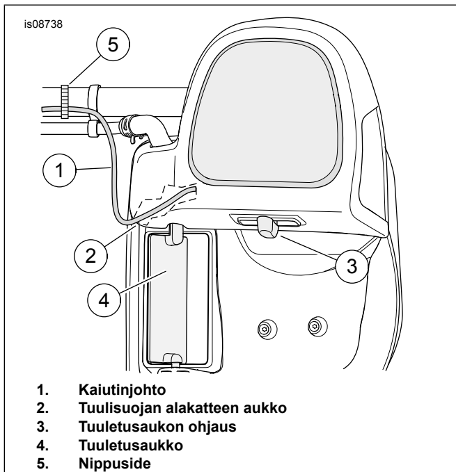
Kuva 1. Kaiutin johtojen reitittäminen
