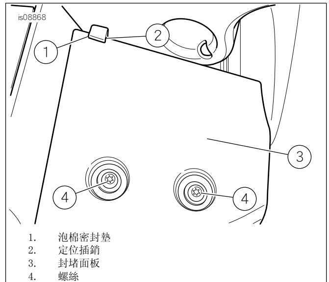
圖9。封堵面板和定位插銷泡棉
