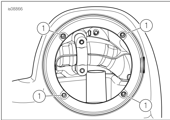
圖11。緊箍螺母
