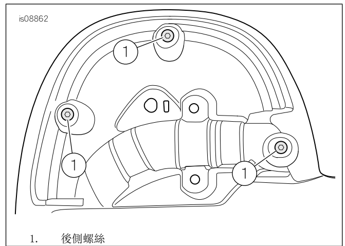
圖8。後側螺絲
