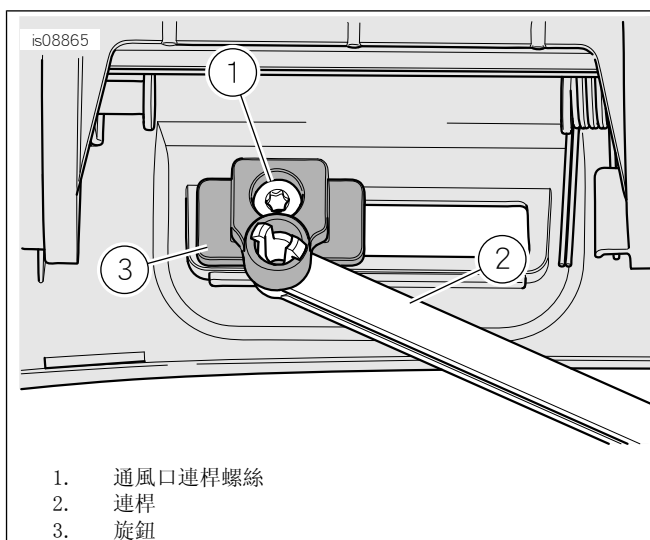
圖4。通風口連桿螺絲
