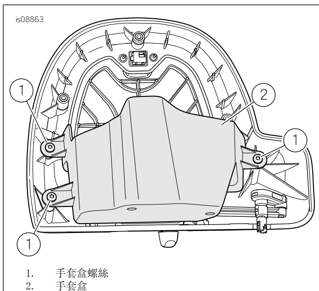
圖3。手套盒螺絲
