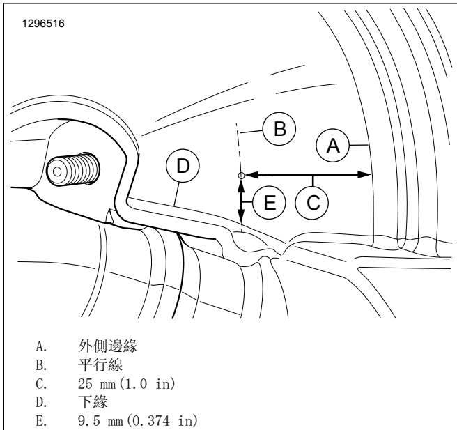
圖10。鑽孔位置
