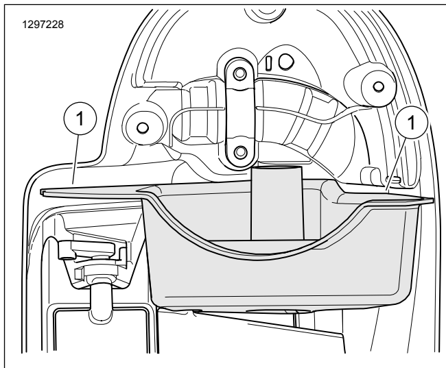
圖5。下方擋風板的密封墊接合表面
