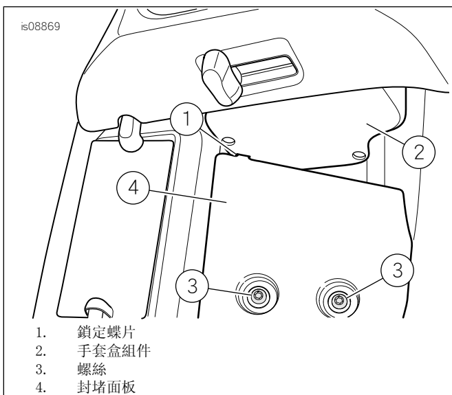
圖2。鎖定插銷和封堵面板
