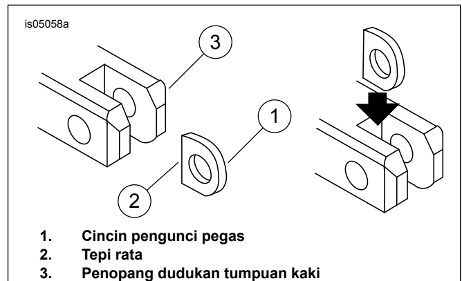
Gambar 1. Pemasangan Cincin Pegas
