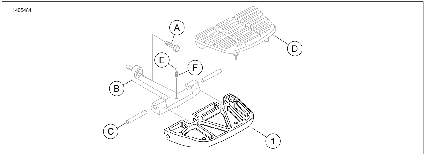
รูปภาพ 1 เนื้อหาเกี่ยวกับชุดอุปกรณ์: ส่วนประกอบชุดอุปกรณ์ฐานแป้นวางเท้าผู้โดยสาร
